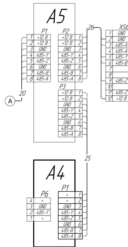
Установка подключения ПДУ
