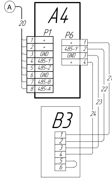
Установка ОПД
