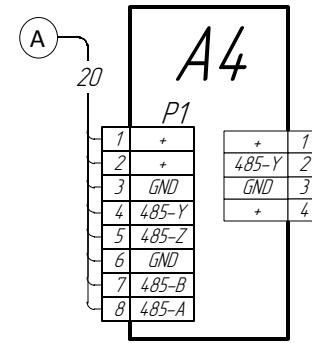
Установка пульта управления
