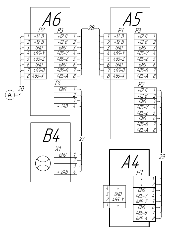
Установка системы КРГ
